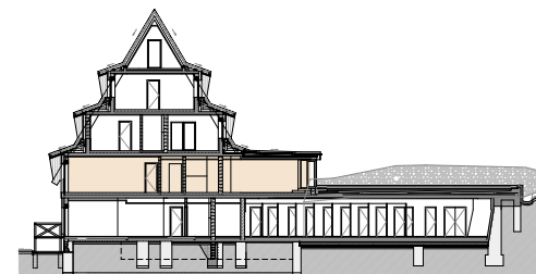
schematický řez
