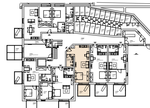
celkový půdorys - umístění na podlaží
